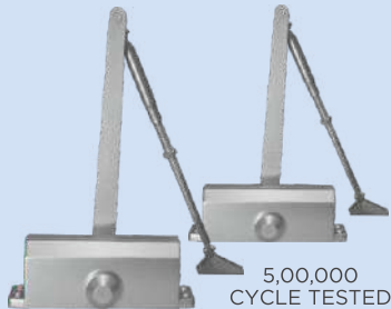
24 DOOR CLOSER - PELMET ARM
